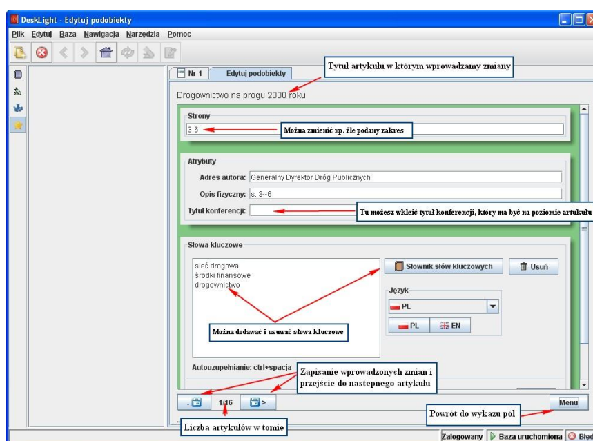
Rys.26. Opis formularza „Edytuj podobiekt”
